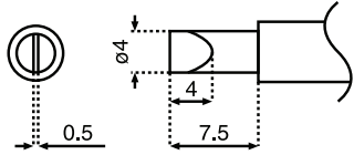
WQD-4D / WQD-4D-C*
